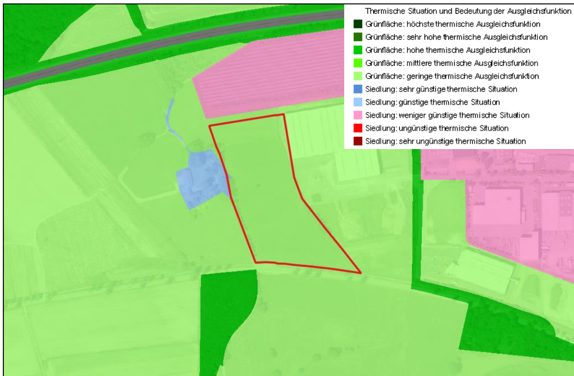
Abbildung 18: Auszug aus der Klimaanalysekarte des LANUV NRW (2023f). Dargestellt ist die Gesamtbetrachtung der Klimaanalyse im Bereich des Plangebietes (rot markiert).
